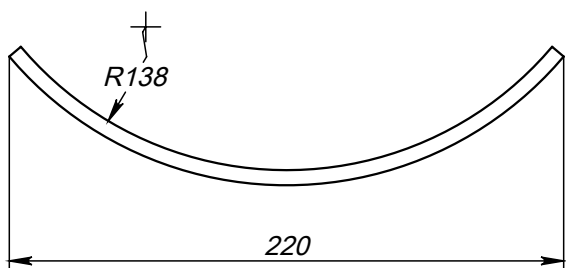
Поз.3 (Ложмент)
